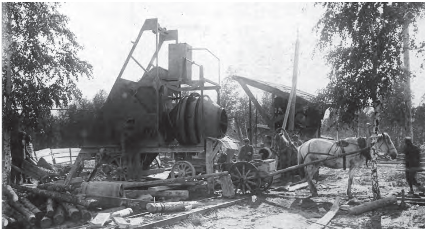
Развозка бетона. 1933 г.
